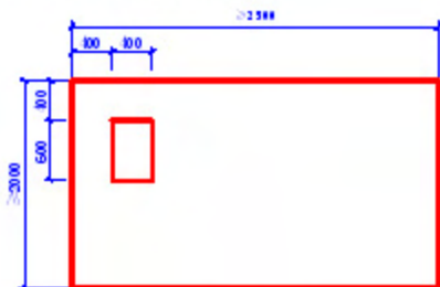
图 A.2.1 试样
