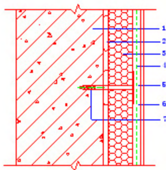
图6.1.1 EPS板薄抹灰系统
