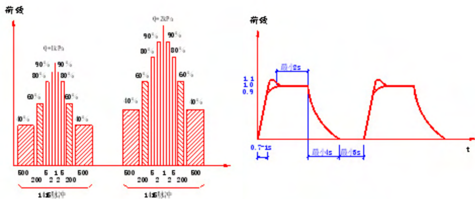
图 A.3.3 加压步骤及压力脉冲图形
