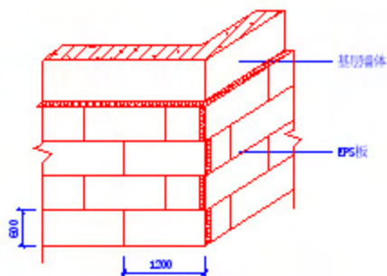
图 6.1.9 (a) EPS 板错缝图
