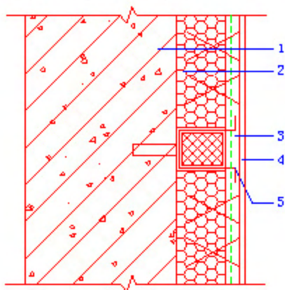
图6.5.1 机械固定系统
