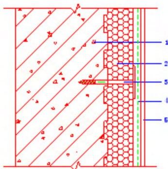
图 6.3.1 无网现浇系统
