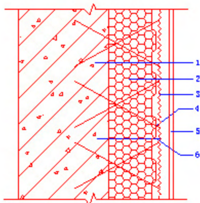
图6.4.1 有网架系统
