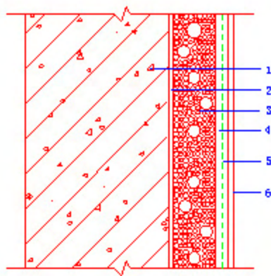
图6.2.1 保温浆料系统
